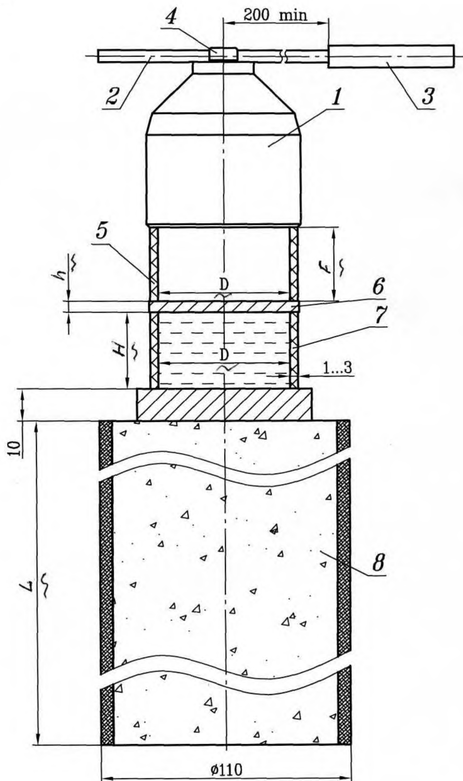
1 – КЗ; 2 – отрезок ДШ; 3 – электродетонатор; 4 – фиксатор (при необходимости); 5 – фокус-дистанционная втулка (пластик); 6 – стальная пластина (сталь Ст3-Ст20, квадрат 50х50); 7 – клиренс-втулка (пластик) с водой; 8 – МКБ
