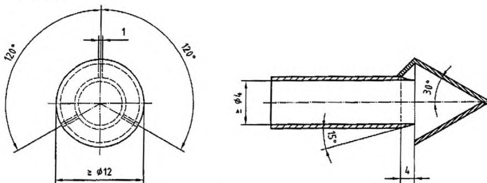
Рисунок 12 – Пробоотборник с коническим наконечником
