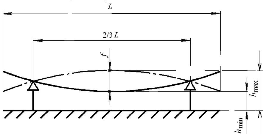
Рисунок 1 – Отклонение трубы от прямолинейности
