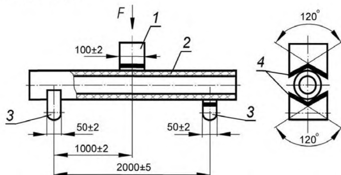
1 – деталь, передающая нагрузку; 2 – образец; 3 – опора; 4 – резиновая прокладка Рисунок 3 – Схема стана для определения прочности труб при изгибе
