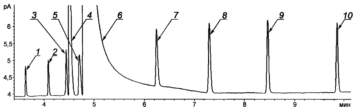
1 — уксусный альдегид; 2 — метилацетат; 3 — этилацетат; 4 — метанол; 5 — 2-пропанол; 6 — этиловый спирт; 7 — 1-пропанол; 8 — изобутиловый спирт; 9 — 1-бутанол; 10 — изоамиловый спирт
