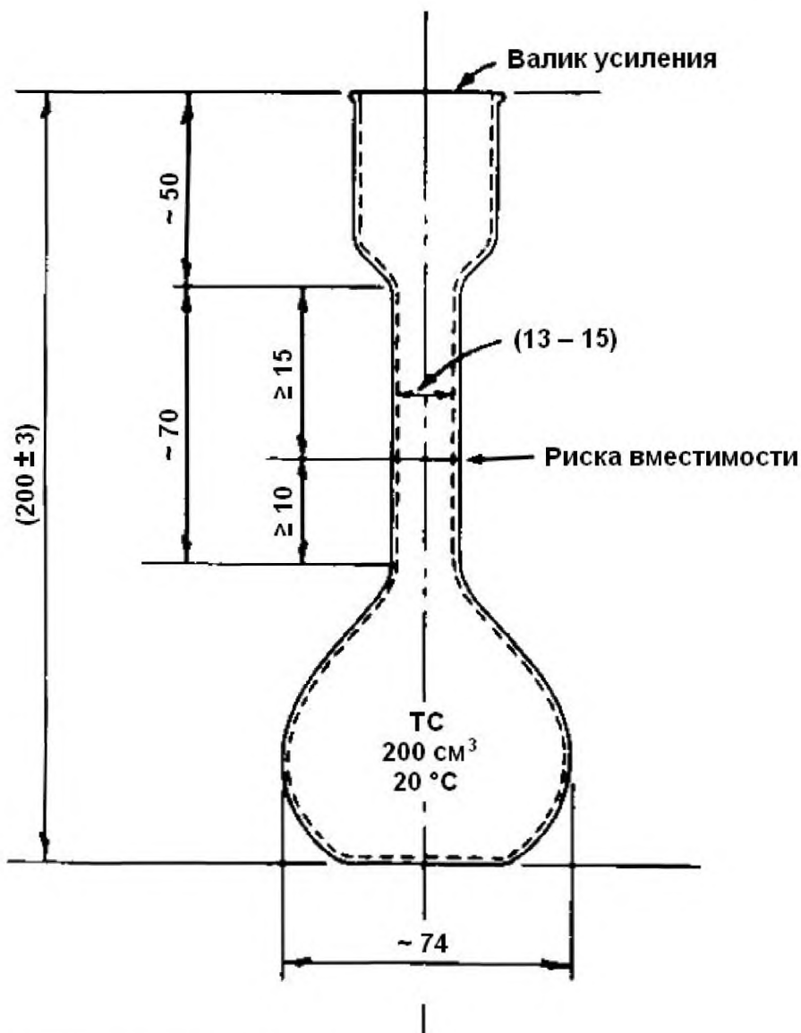
Рисунок 3 – Колба Кольрауша
