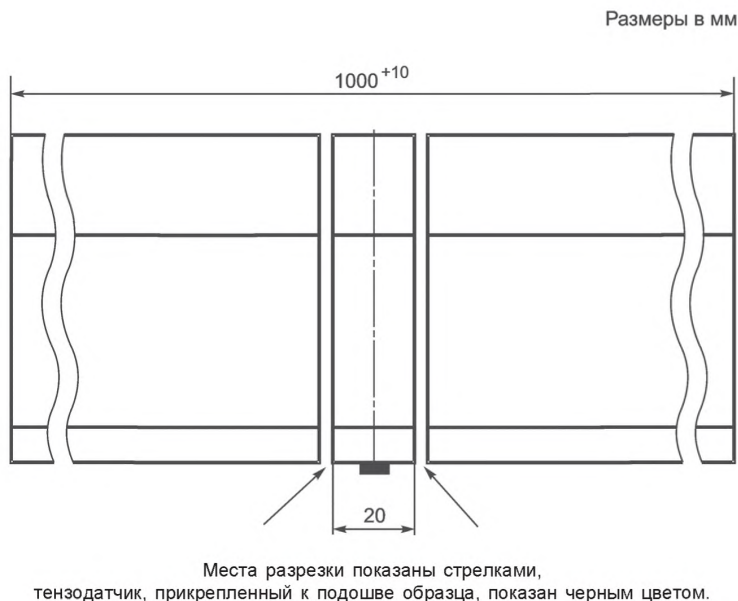
Рисунок 14 — Схема разрезки образца при определении остаточных напряжений в подошве рельса
