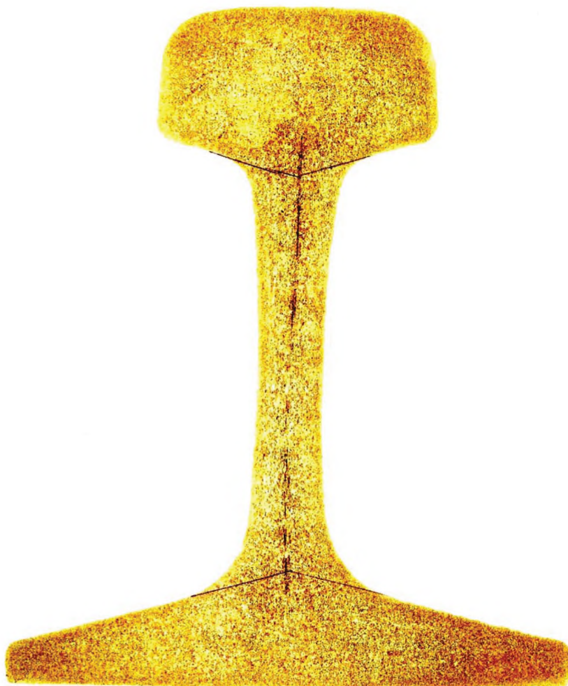
Рисунок И.5 — Осевая ликвация в шейке, простирающаяся в головку и (или) в подшву (серный отпечаток)
