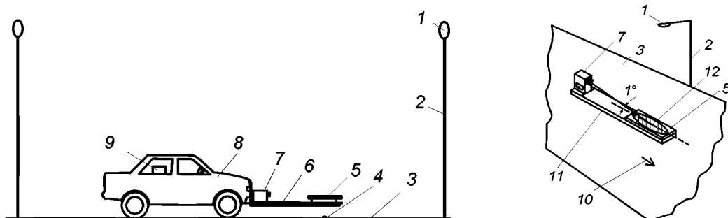
а) мобильный способ 1 – светильник; 2 – опора; 3 – покрытие контрольного участка; 4 – точка измерения; 5 – тест-образец покрытия; 6 – консоль; 7 – яркомер; 8 – автомобиль; 9 – устройство управления; 10 – направление движения; 11 – общее основание измерительного устройства; 12 – измерительное поле яркомера (заштриховано) б) стационарный способ
