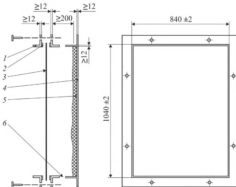
1 – стальная зажимающая рама; 2 – резиновые полосы; 3 – испытываемый образец; 4 – стальной приемный ящик; 5 – амортизирующий материал; 6 – вентилируемые отверстия Рисунок 1 – Пример оборудования для крепления образца
