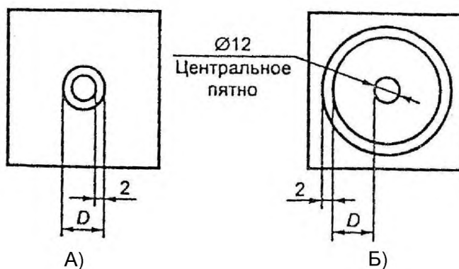
Рисунок 7.6 – Формы мишеней
