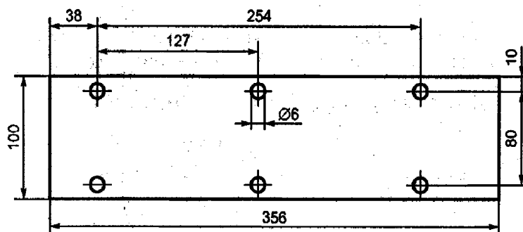
Рисунок 7.22 — Испытуемый образец
