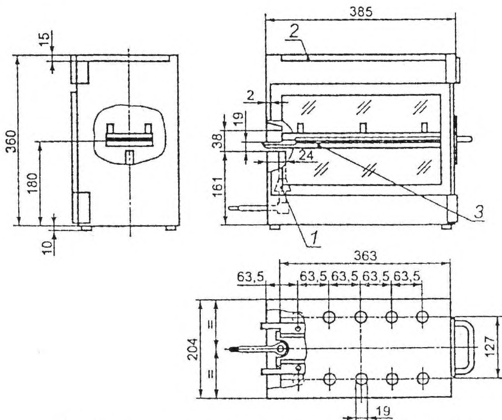
1 — газовая горелка; 2 — вентиляционная щель; 3 — испытуемый образец
