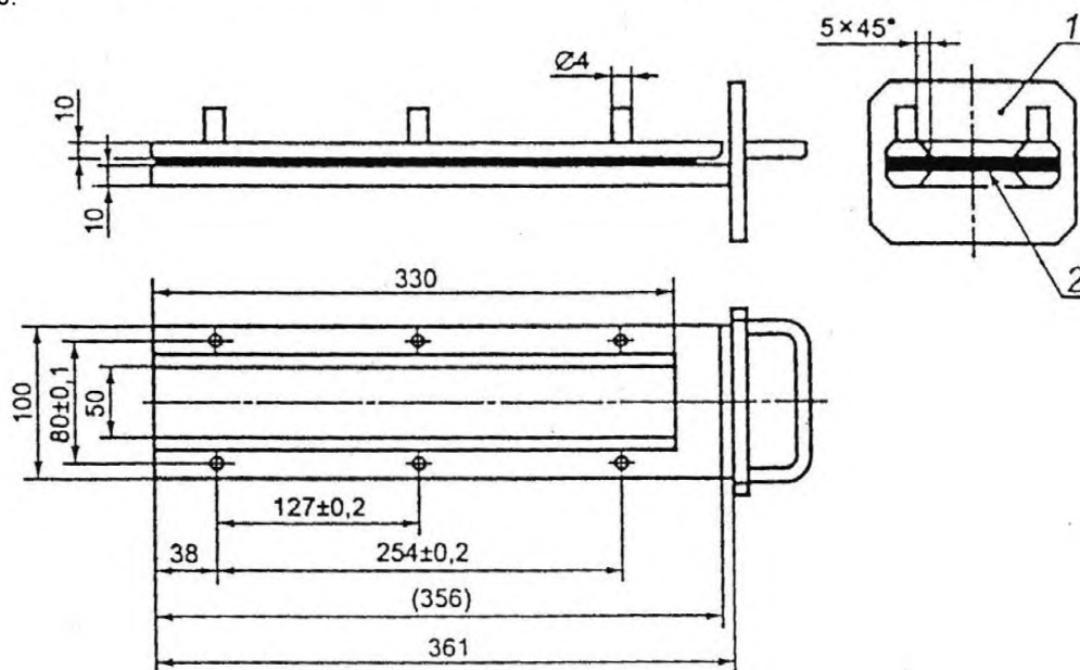
Рисунок 7.20 — Схема подставки
