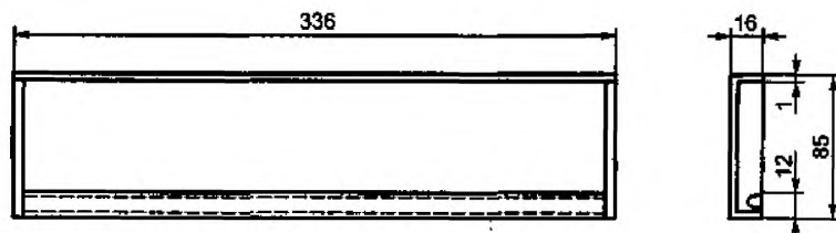
Рисунок 7.19 — Ванночка
