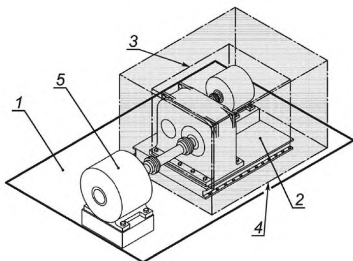
Рисунок 1 — Огибающий параллелепипед и измерительная поверхность для редуктора
