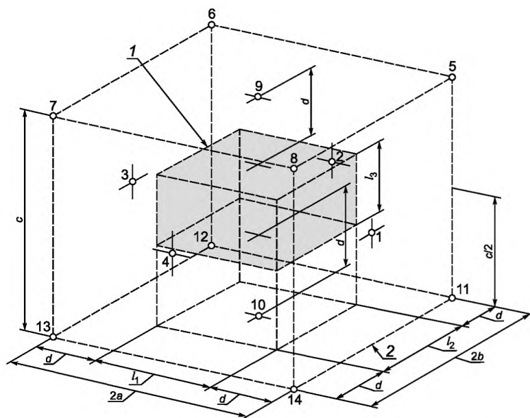
1 — огибающий параллелепипед; 2 — измерительная поверхность
