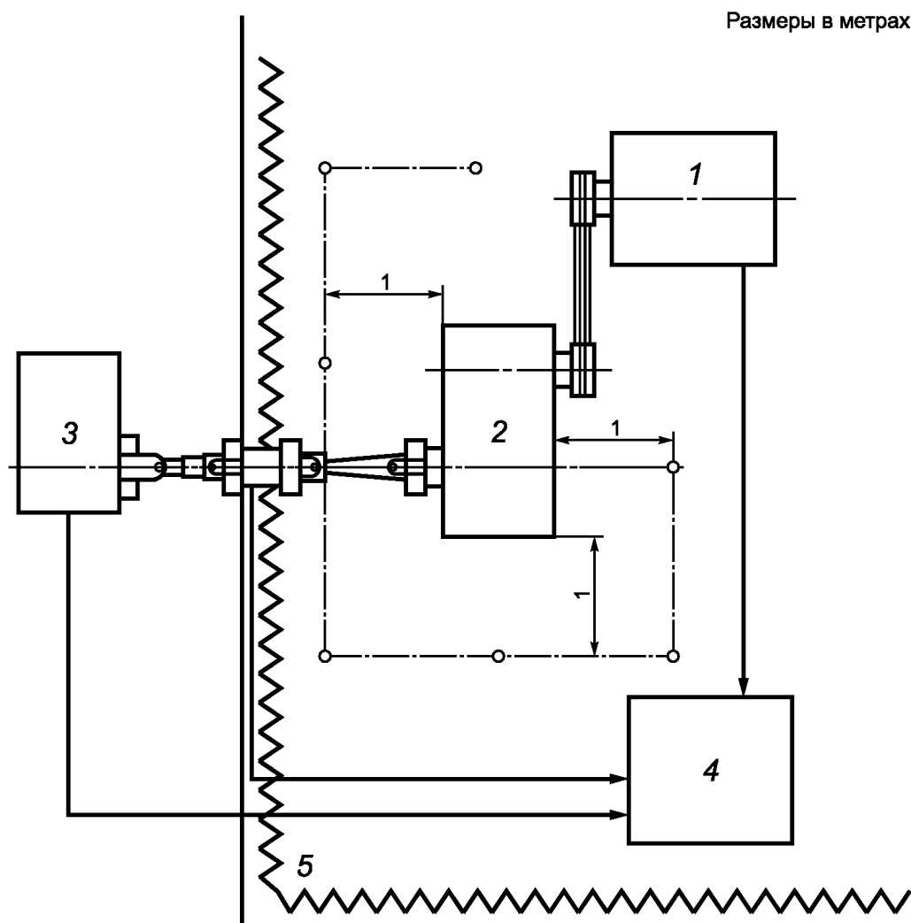
Рисунок А.7 — Типовая испытательная установка на месте эксплуатации для определения уровней шума составных частей
