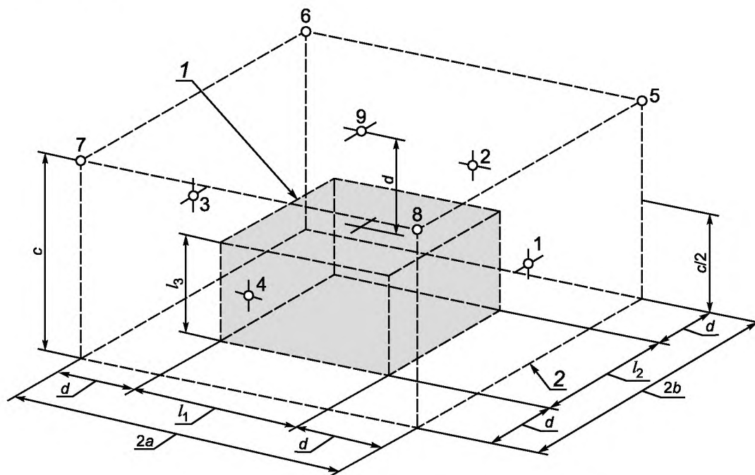
1 — огибающий параллелепипед; 2 — измерительная поверхность
