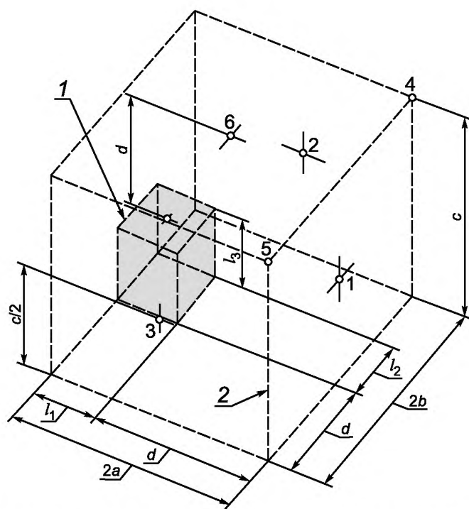
1 — огибающий параллелепипед; 2 — измерительная поверхность
