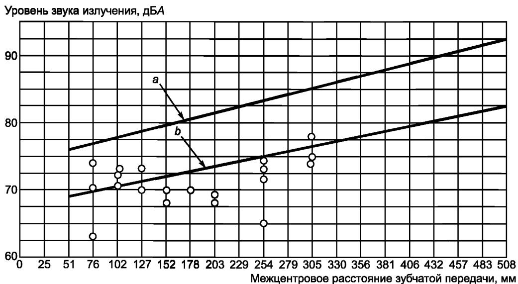
Рисунок В.6 — Приращение уровня звука излучения \Delta L_{pA} относительно уровня на холостом ходу в зависимости от P/P_R
