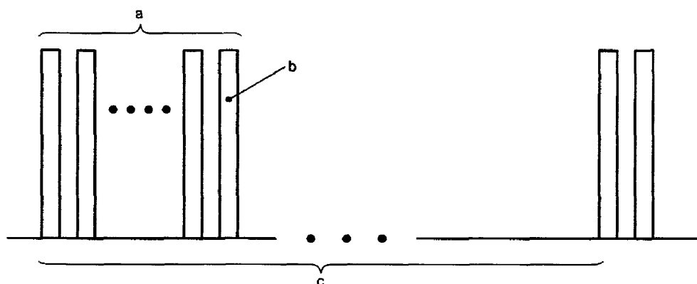
Рисунок 7 – Радиointерфейс DSSS
