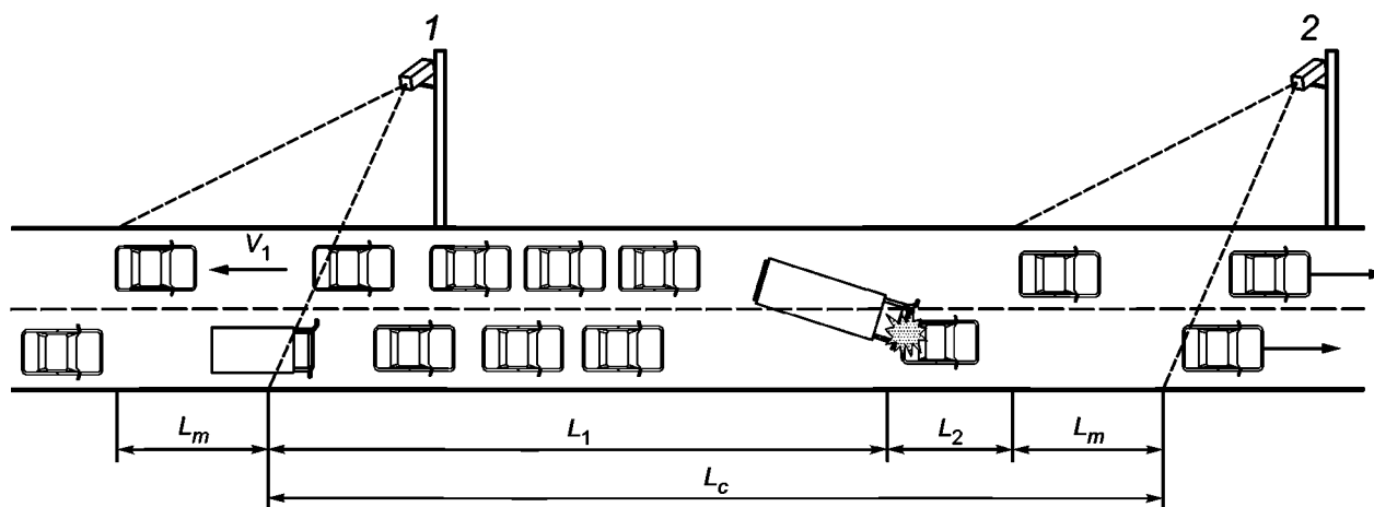
1 — положение камеры A; 2 — положение камеры B; L_c — интервал между положениями камер; L_m — зона покрытия камеры; V_1 — скорость распространения затора
