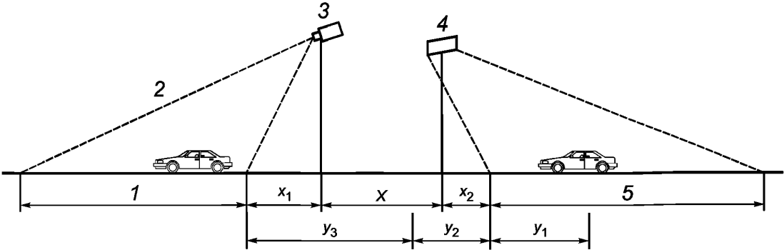
1 — зона покрытия камеры наблюдения; 2 — место возникновения затора; 3 — камера наблюдения; 4 — информационное табло; 5 — зона, в которой возможно распознавание сообщения на табло; X — определяемое расстояние между местами установки камеры и табло; x_1 — слепая зона камеры; x_2 — предел видимости информационного табло; y_1 — дистанция принятия решения; y_2 — дистанция реакции водителя; y_3 — тормозной путь
