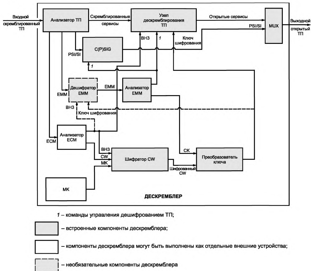
Рисунок 2 — Структурная схема МОД
