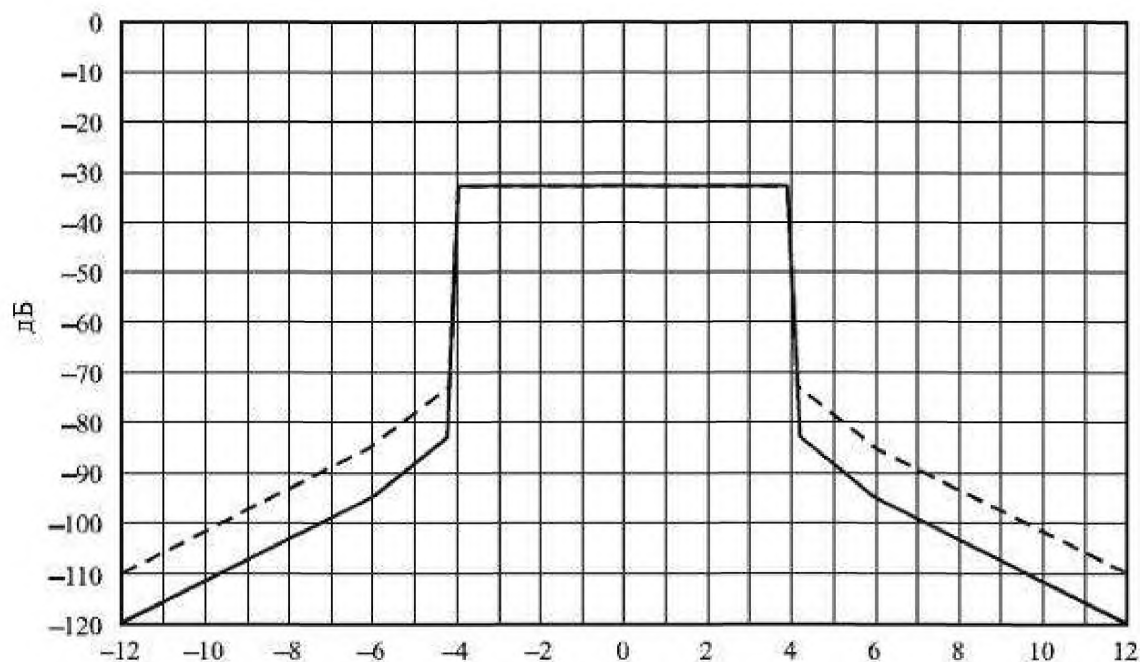
Частота относительно средней частоты полосы частот радиоканала, МГц Уровень мощности, измеренной в полосе 4 кГц, где 0 дБ соответствует общей выходной мощности — — — Стандартная спектральная маска ————— Критическая спектральная маска
