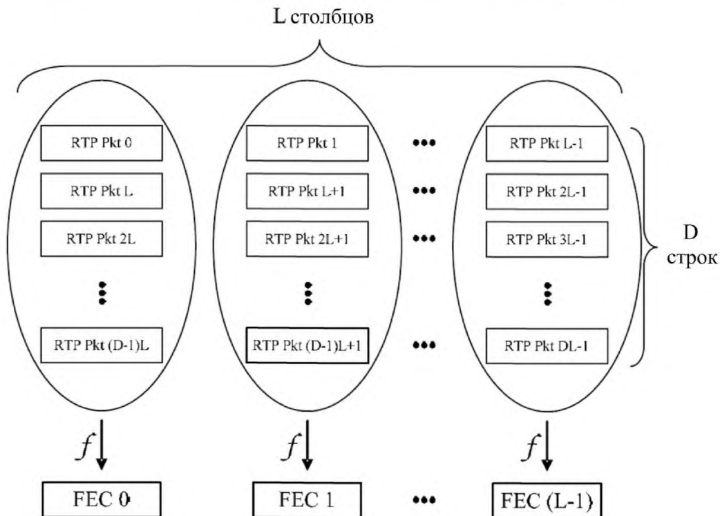
Рисунок 1 – Схема организации защищаемых пакетов
