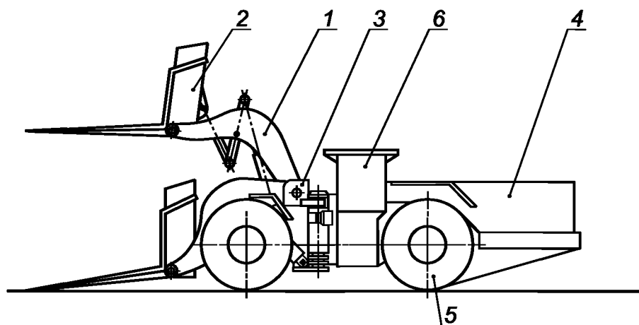
1 — манипуляционное устройство; 2 — монтажная платформа; 3 — шарнирно сочлененная рама; 4 — дизельный привод; 5 — ходовая часть; 6 — кабина машиниста
