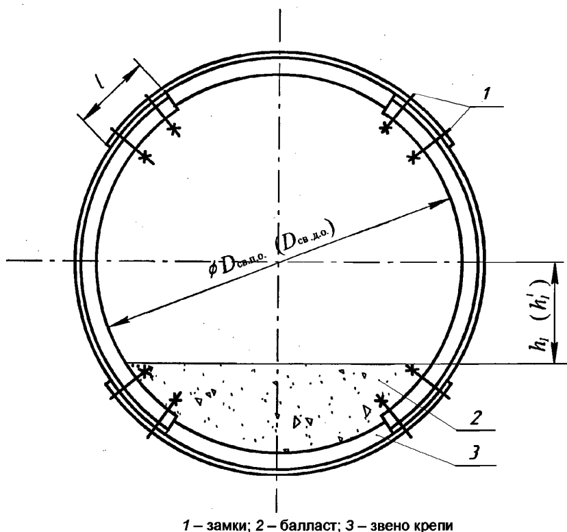
Рисунок 1 – Схема кольцевой крепи
