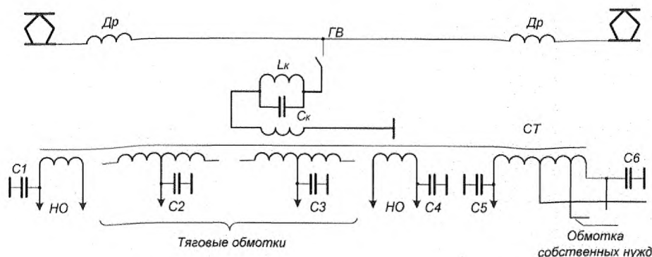
Рисунок 7.2 - Схема подавления помех для ЭПС переменного тока
