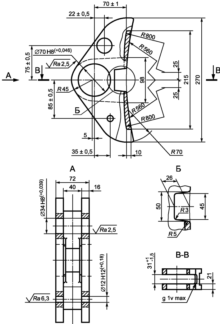
Рисунок 10 — Башмак типа 5
