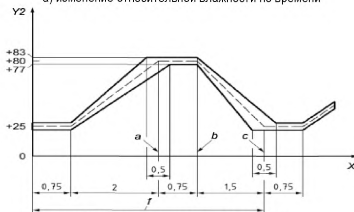
b) изменение температуры по времени
