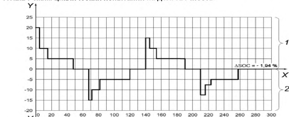
Рисунок 7 — Изменение тока по времени в режиме постепенного разряда для циклического испытания на долговечность
