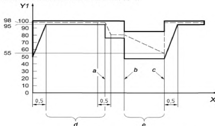
a) изменение относительной влажности по времени
