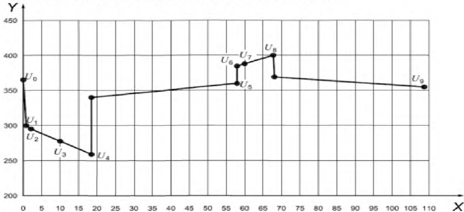
X – время, с; Y – напряжение батарейного блока или батарейной системы (в качестве примера), В. Рисунок 6 — Снятие характеристик мощности в импульсе (график по напряжению).
