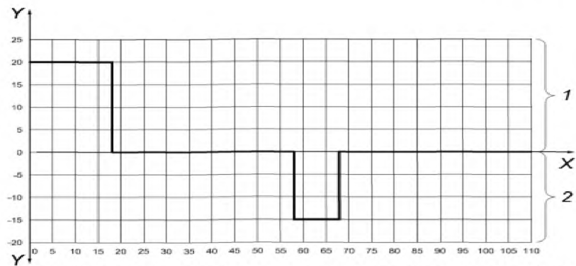
X – время, с; Y – ток (измеряемый в величинах, кратных С); 1 – разряд; 2 – зарядка Рисунок 5 — Снятие характеристик мощности в импульсе (график по току)
