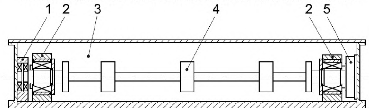
1 – осевой АМП; 2 – радиальный АМП; 3 – вакуумная камера; 4 – ротор; 5 – двигатель
