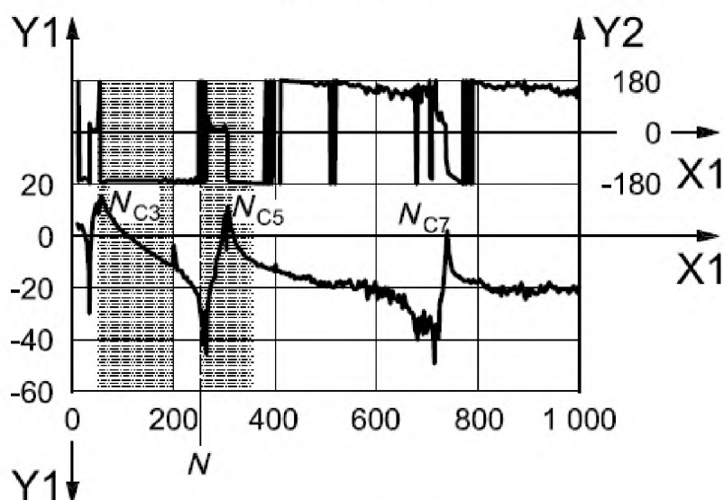
а) Диаграмма Бode передаточной функции разомкнутой цепи G_o
