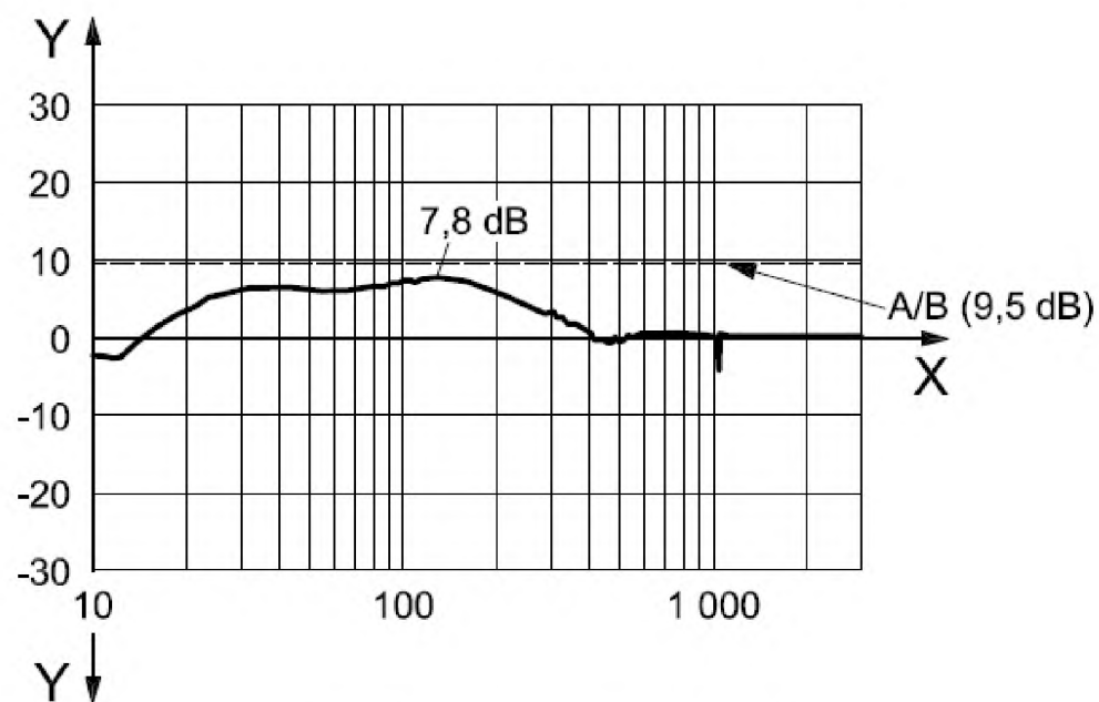
Рисунок С.3 – Функция чувствительности G_s ротора NEDO
