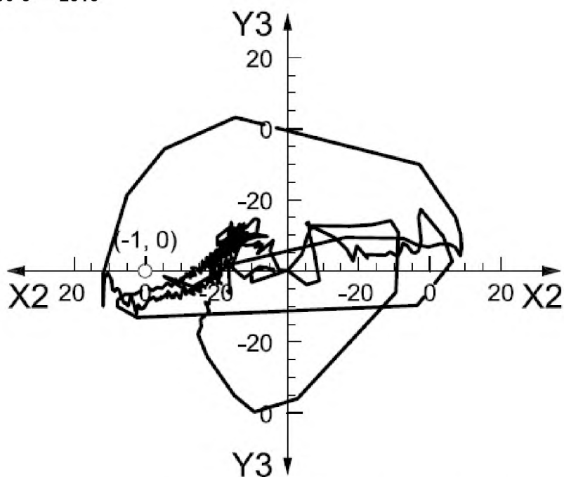
б) Диаграмма Найквиста передаточной функции разомкнутой цепи G_o
