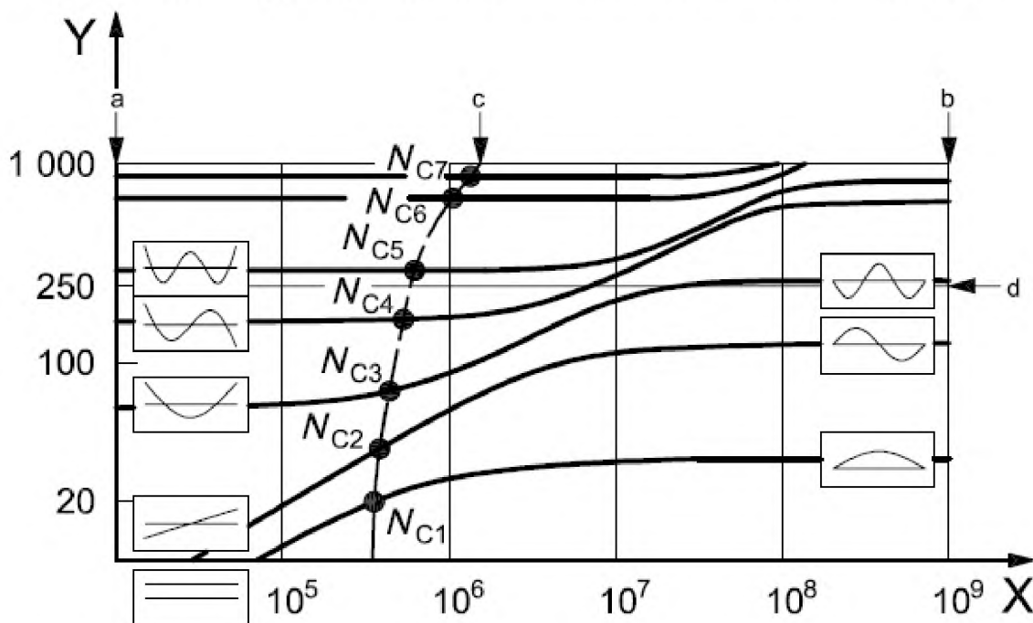
X – жесткость, Н/м; Y – частота, Гц; а – свободные концы ротора; b – заземленные концы ротора; с – жесткость АМП; d – номинальная частота вращения
