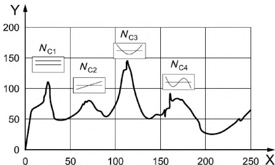
Рисунок А.10 – Изменение вибрации с изменением частоты вращения ротора
