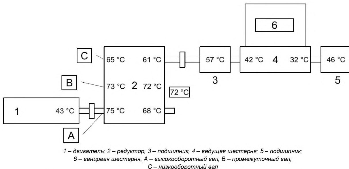
Рисунок С.2 – Результаты измерений температуры на схеме механизма привода шаровой мельницы
