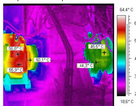
Рисунок С.7 – Корпуса подшипников шестерни привода мельницы
