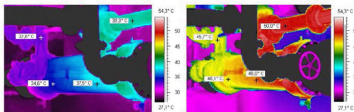
Рисунок С.10 – Термограммы двух маслоохладителей
