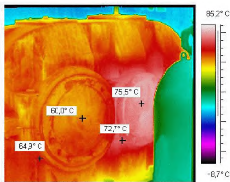
Рисунок С.5 – Редуктор со стороны двигателя
