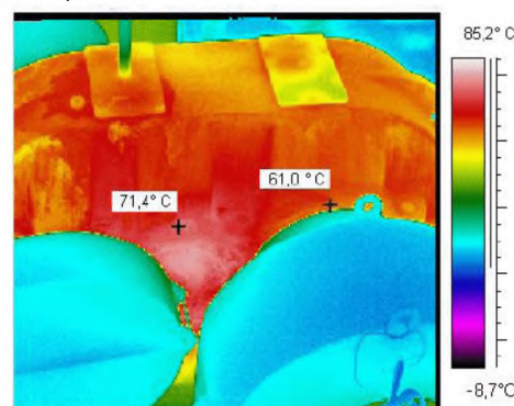
Рисунок С.6 – Редуктор со стороны мельницы
