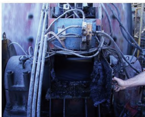
Рисунок С.8 – Ведущая шестерня привода мельницы
