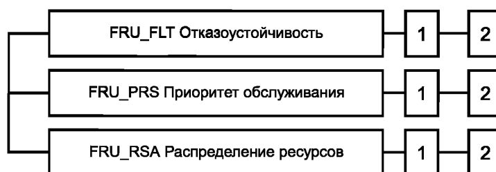
Рисунок К.1 — Декомпозиция класса FRU «Использование ресурсов»
