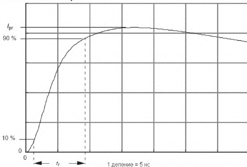
Рисунок 3 – Типичный импульс тока через резистор 500 Ом
