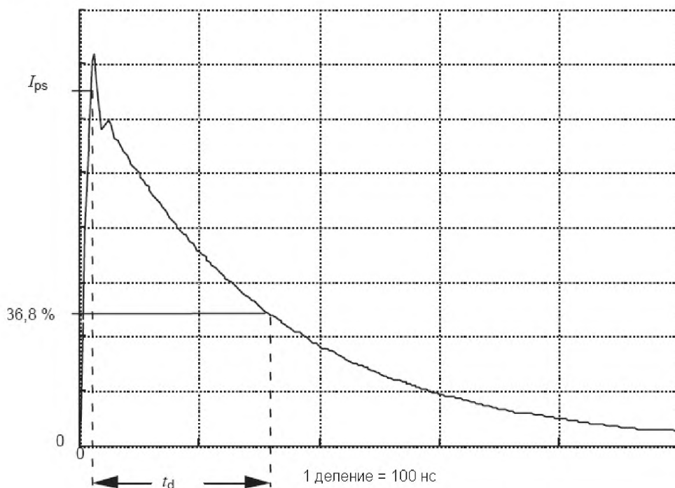
Рисунок 2b – Типичный импульс тока через закорачивающий провод t_d
