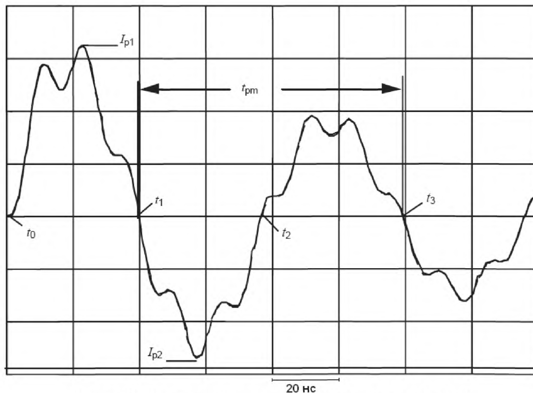
Рисунок 2 – Типичный импульс тока через закорачивающий провод
