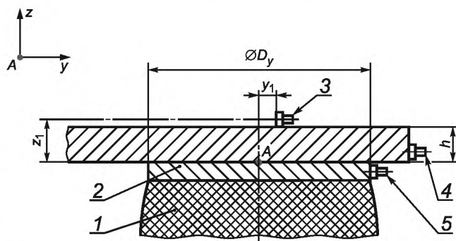
Рисунок 5 — Возможные положения акселерометра для измерений v_y
