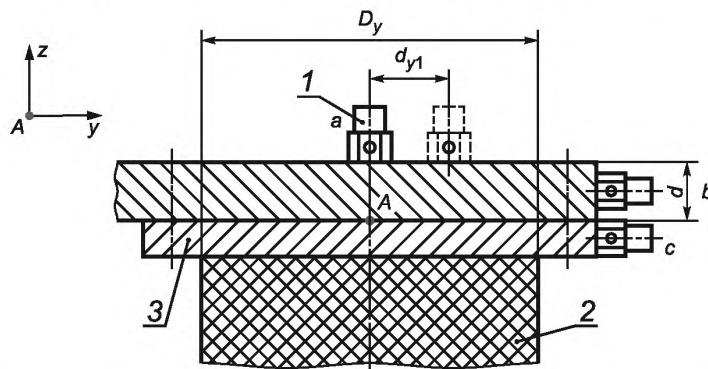
1 — акселерометр; 2 — изолятор; 3 — установочный фланец изолятора; а — точка 1; b — точка 2; с — точка 3
