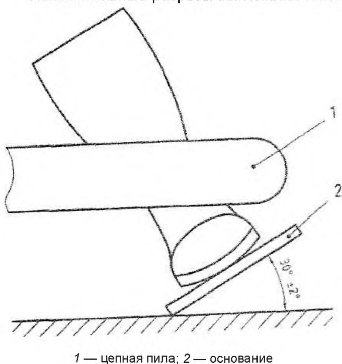
Рисунок 4 — Схема испытания в области союзки
