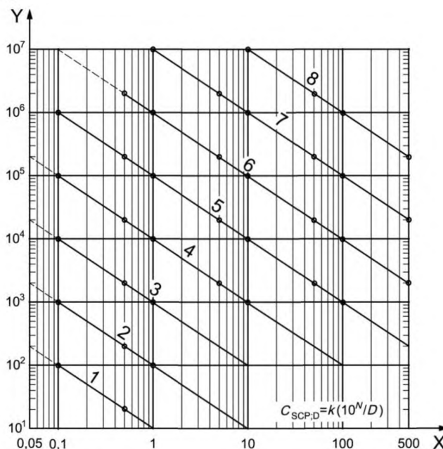
Рисунок 1 – Классы SCP
