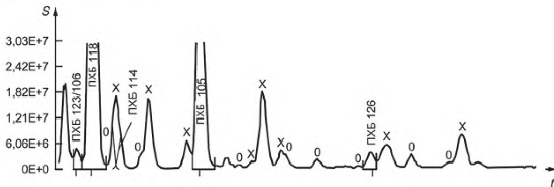
б) ПеХБ [ m/z : 325,881 (100 %)]
