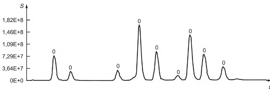
с) ГпХБ [ m/z : 393,802 (100 %)]
