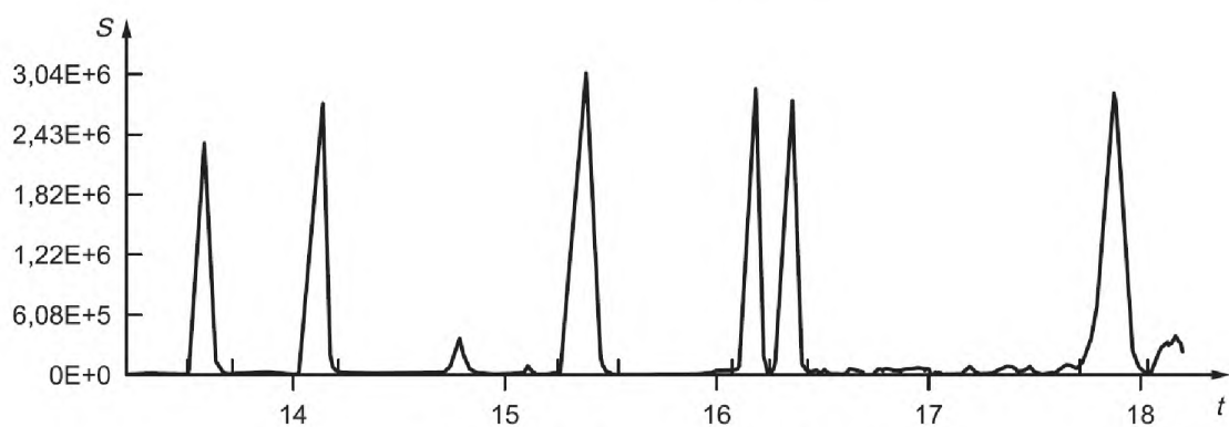
b) ^{13}\text{C}_{12} -ГХБ [ m/z : 371,882 (100 %)]
