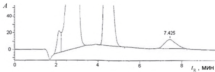
Рисунок В.4 – Хроматограмма, полученная на УФ детекторе при длине волны \lambda = 242 нм для МР-производного 2,4-TDI
