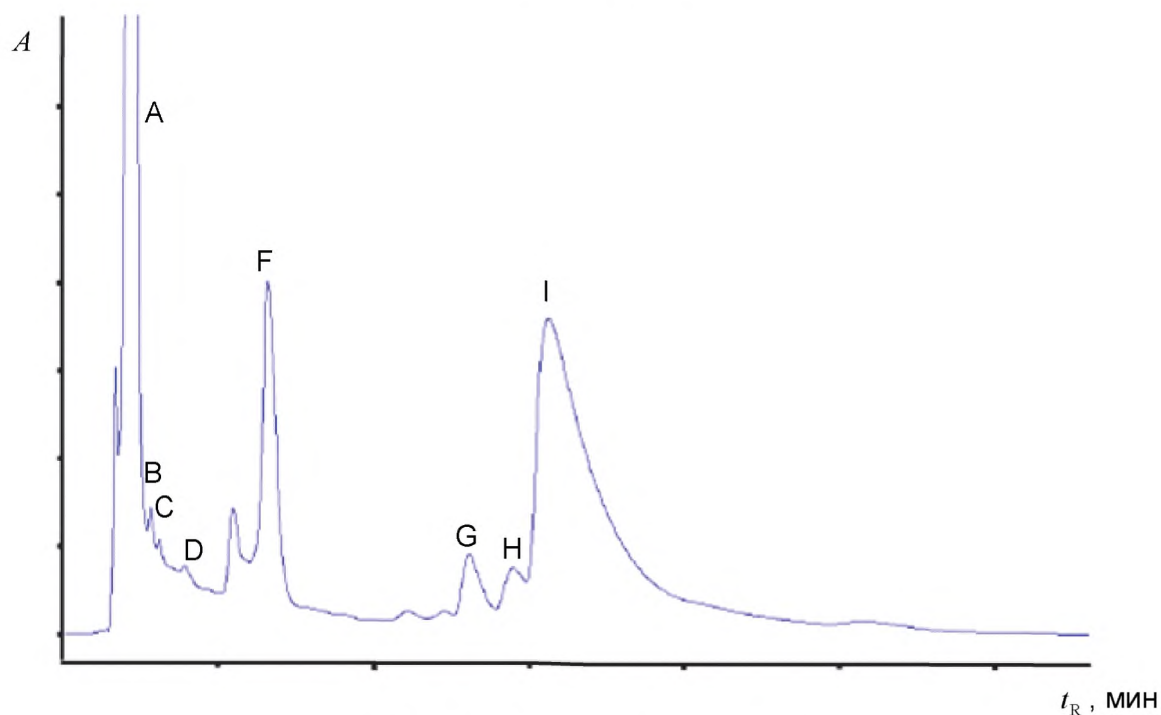
Рисунок В.4 – Хроматограмма, полученная на УФ детекторе при длине волны \lambda = 242 нм для МР-производного 2,4-TDI
