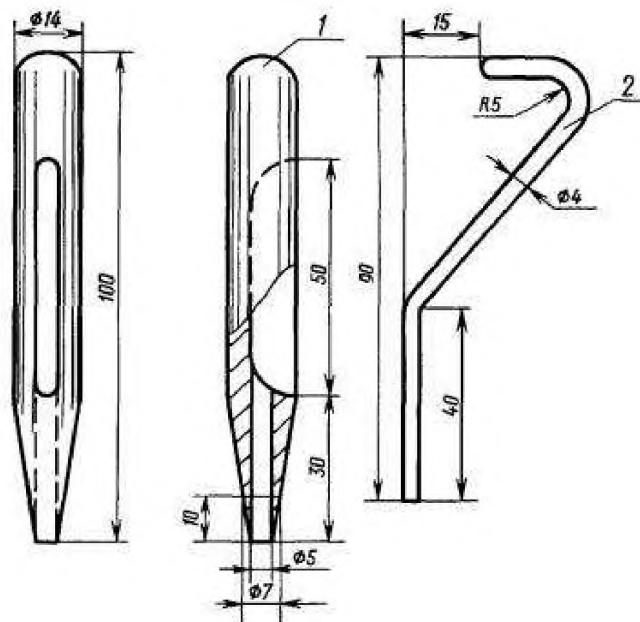
1 - прободоотборник; 2 - поршень
