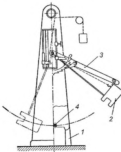
1 – стойки; 2 – маятник; 3 – подъемная рама; 4 – образец
