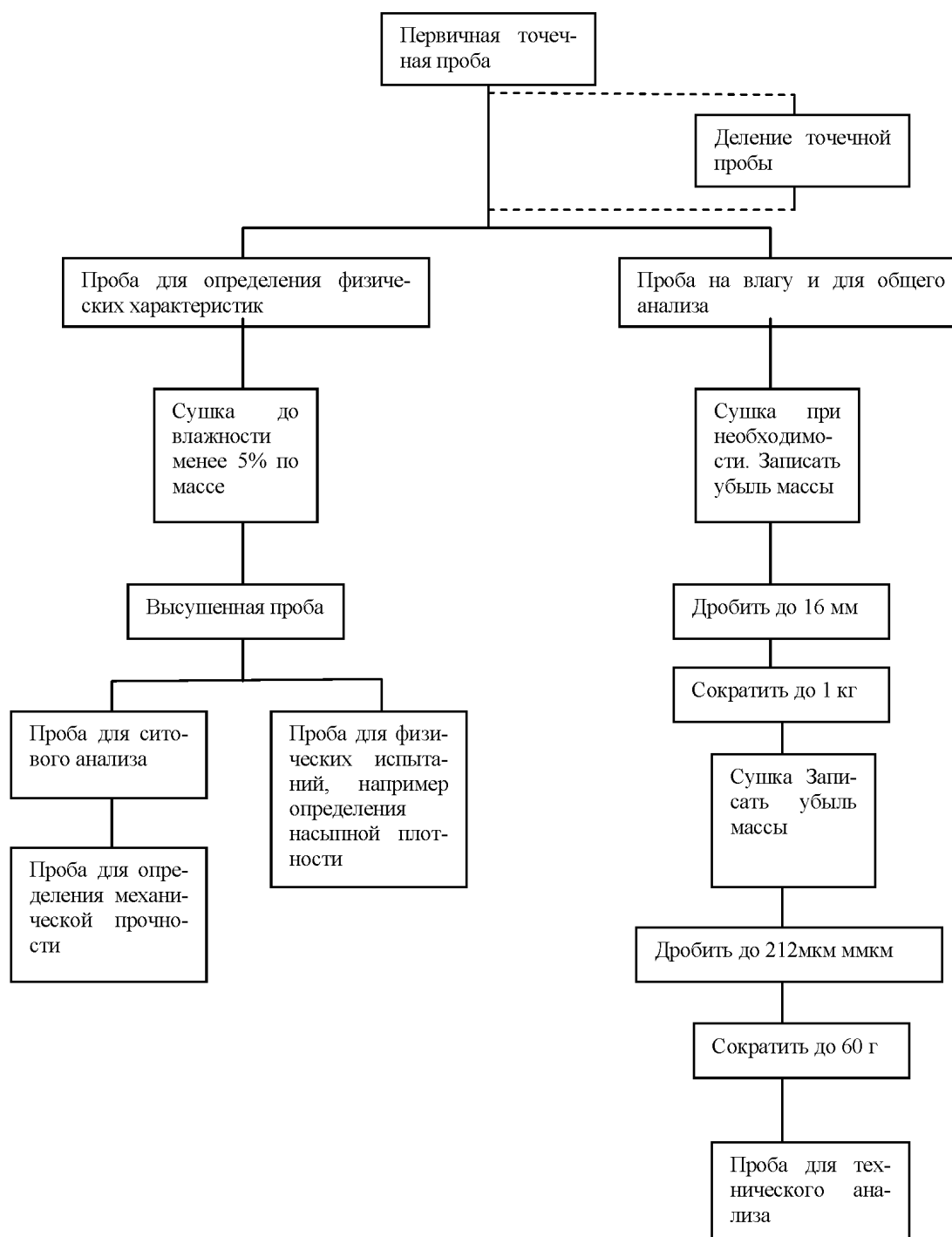
Рисунок 6 – Составление и подготовка проб
