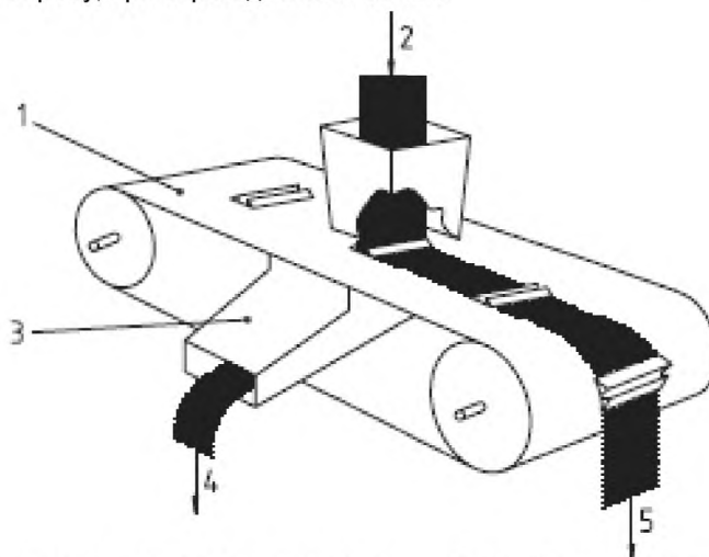
1 — лента со щелями; 2 — подача кокса; 3 — наклонный желоб; 4 — сокращенная проба; 5 — отвал. d) Тип ленточный со щелями.
