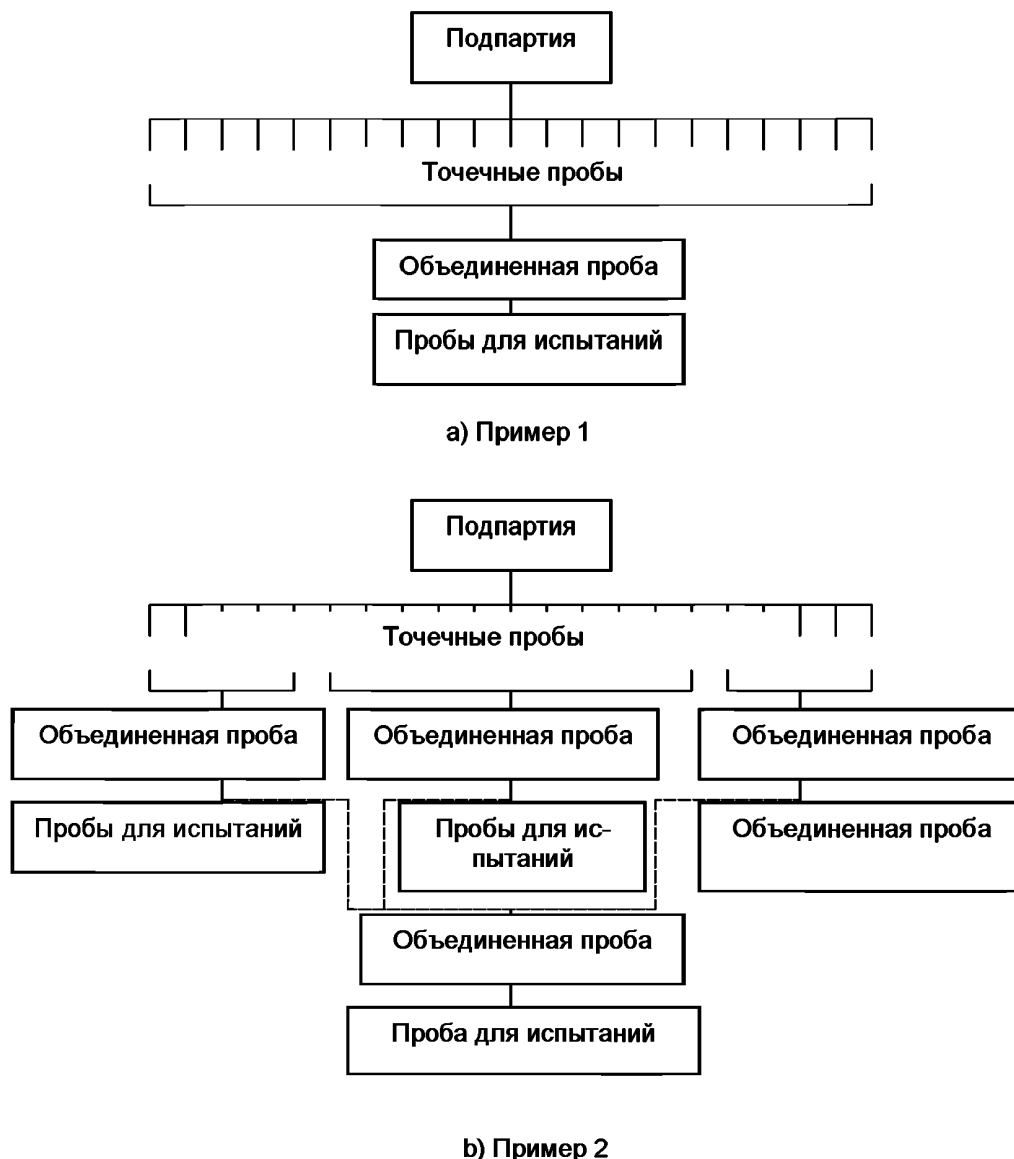
Рисунок 1 — Схемы составления проб
