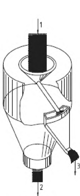
1 —подача кокса; 2 — отвал; 3 — сокращенная проба е) Тип с вращающимся желобом
