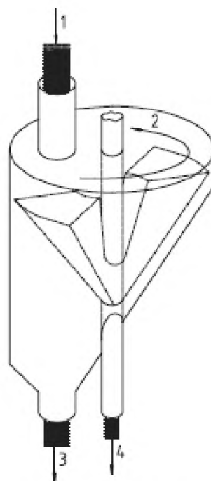
1 — подача кокса; 2 — вращающийся бункер; 3 — отвал; 4 — сокращенная проба ф) Тип вращающийся бункер и труба.
