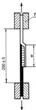
1 – зажим; w – ширина клеевого соединения
