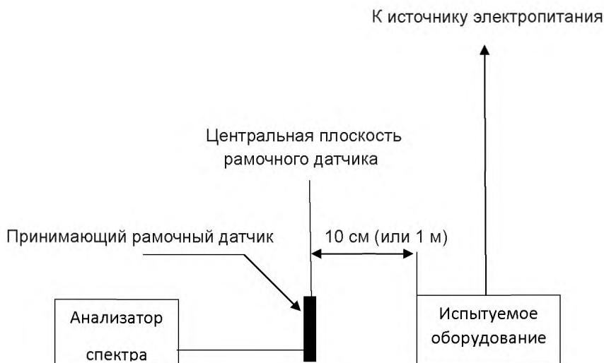
Рисунок А.2 - Испытательная установка для измерения магнитного поля, в полосе частот 50 Гц-50 кГц
