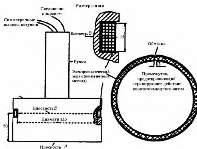
Рисунок А.1 - Конструкция рамочного датчика
