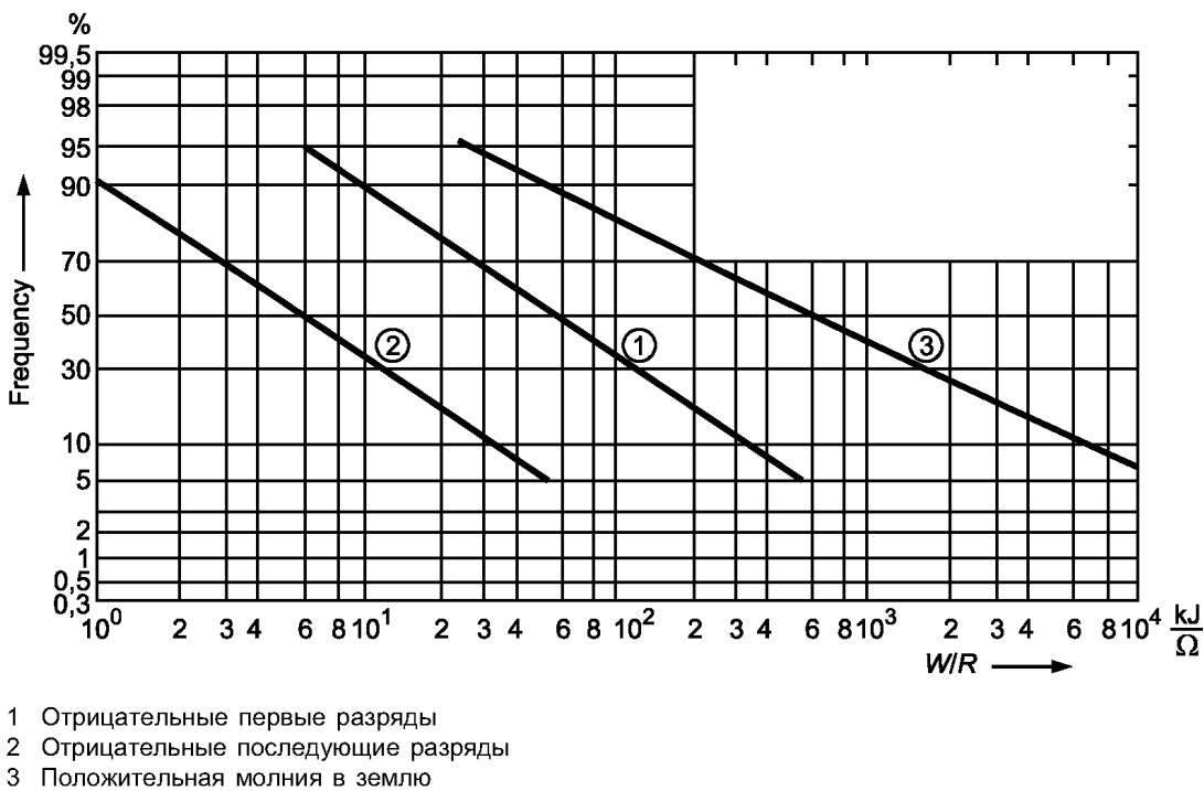
Рисунок А.4 — Частотное распределение энергии молнии W/R
