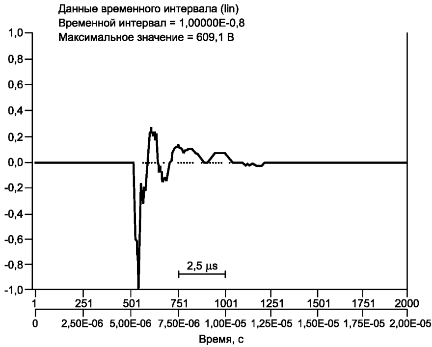
Рисунок 15 — Пример высокочастотного импульса коммутационного перенапряжения
