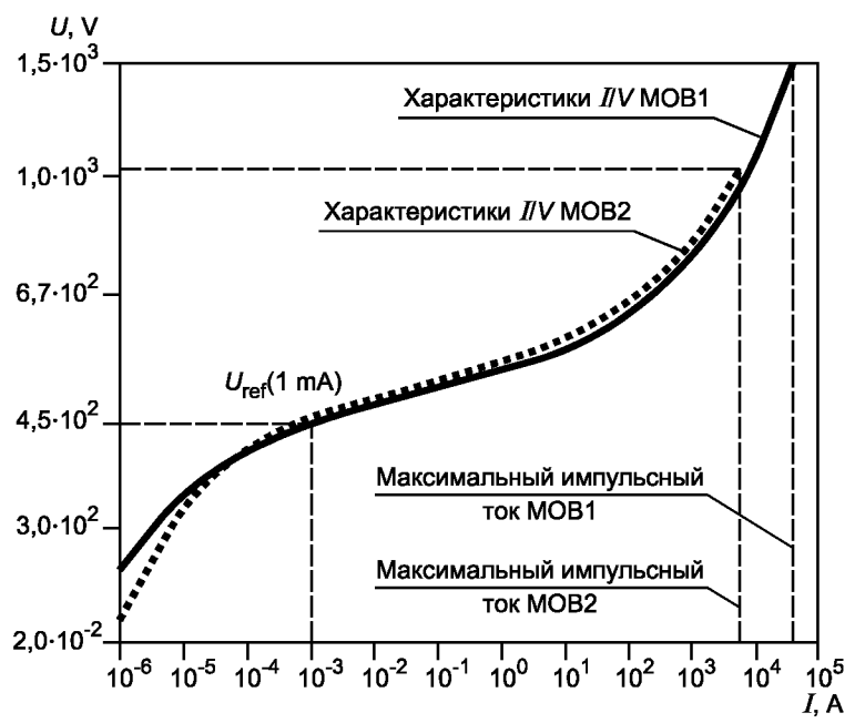
Рисунок Е.2 — Сравнение вольтамперных характеристик двух МОВ
