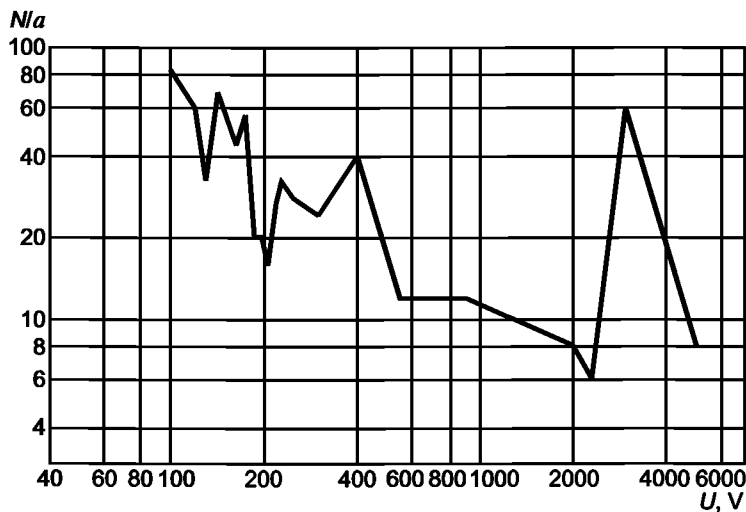
Рисунок В.7 — Коммутационные импульсные перенапряжения на промышленном предприятии, измеренные вблизи распредустройства
