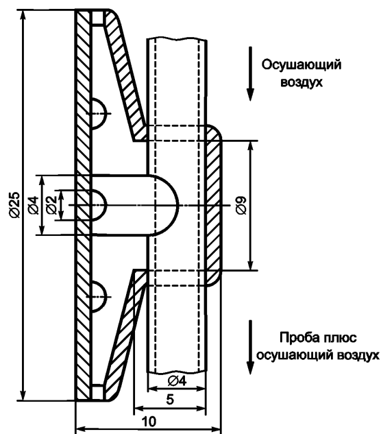
Рисунок 9 — Пробоотборник
