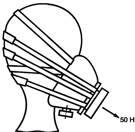
Рисунок 1 — Размещение соединительного узла при испытании
