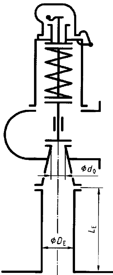
Рисунок 4.1 – Предохранительные клапаны
