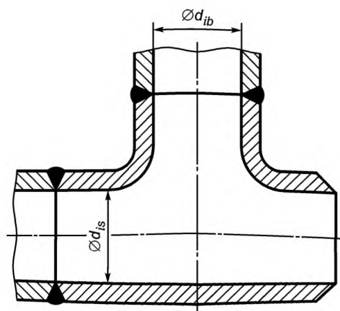
Рисунок 8.1-5 — Ковано-штампованный штуцер
