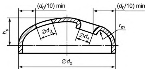
Рисунок 10.2-5 — Отверстия в днищах
