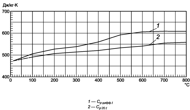
Рисунок D-3c — Теплоемкость сталей групп 8.2 и 215S15
