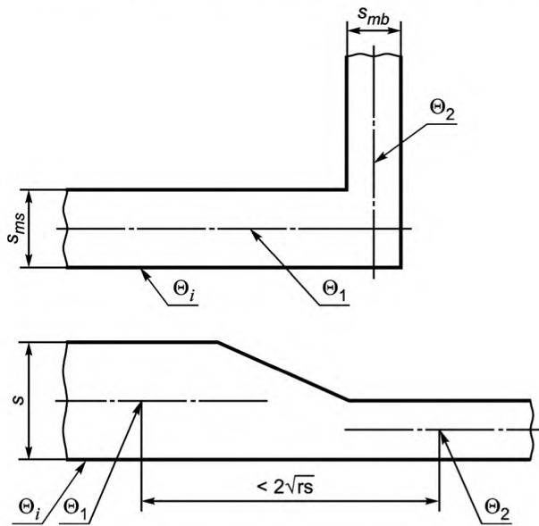
Рисунок 13.3-1 – Определение \Delta\Theta
