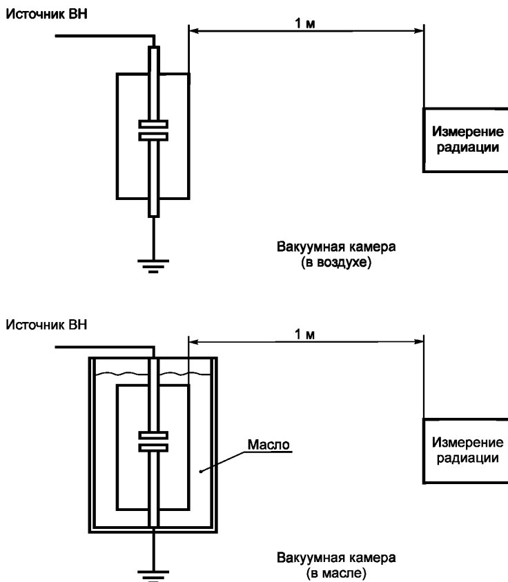
Рисунок 3 — Расположение дозиметра при испытаниях
