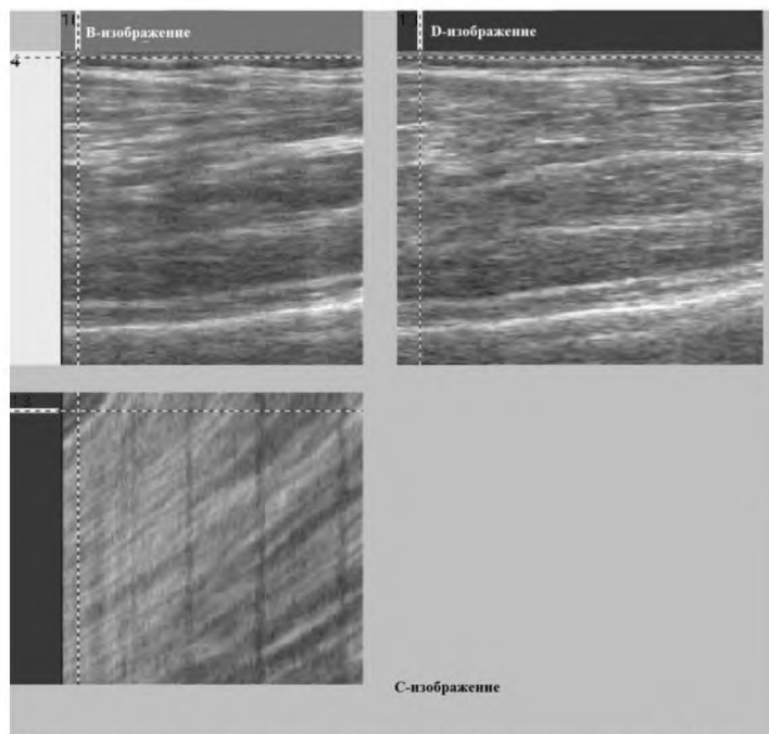
Рисунок D.2a) В-, D-, С- изображение и фиксированный образ на С-изображении
