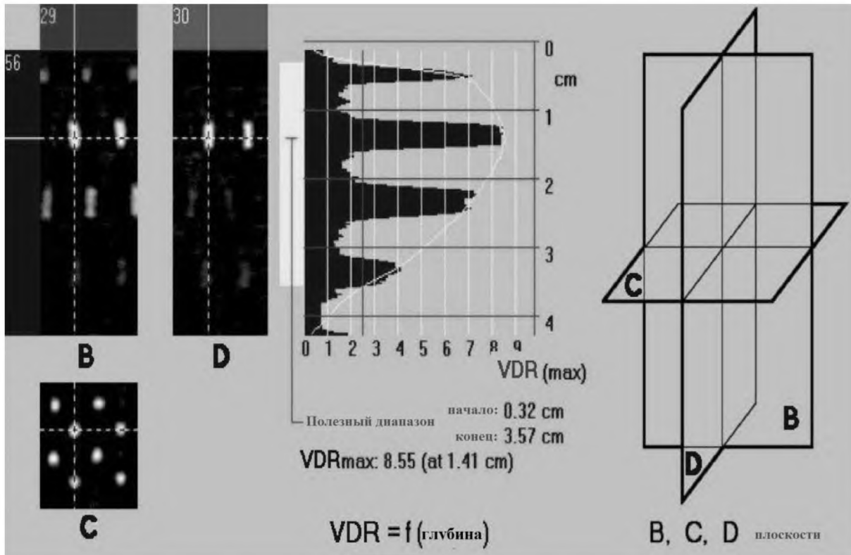
Рисунок А.12 Схематическое изображение B-, D-, C- плоскостей
