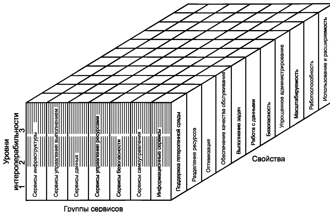
Рисунок 2 — Модель СОАОГС
