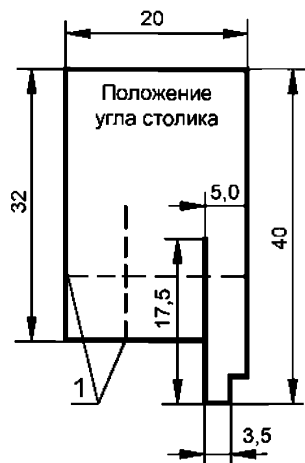
Рисунок 1 – Форма и размер образца для испытания
