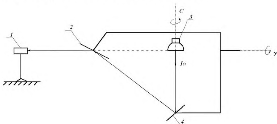
1 – фотометрическая головка; 2, 4 – зеркала; 3 – ОП или ИС; I_o – осевая сила света; C – ось вращения плоскостей C (поворот ОП); \gamma – угол поворота зеркал 2, 4
