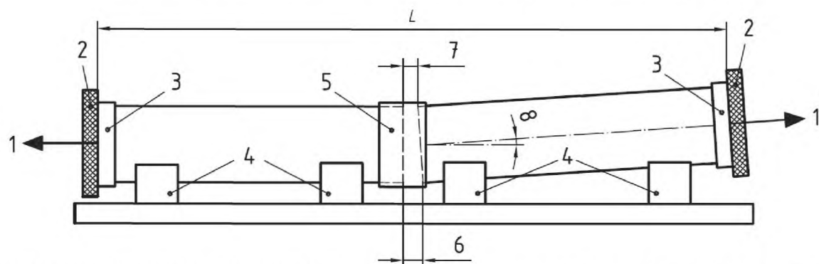
1 – осевое давление, воздействующее на образец; 2 – оснастка испытательного стенда; 3 – торцевая заглушка; 4 – опоры; 5 – испытуемое соединение; 6 – общий вырыв; 7 – хомут; 8 – угловое смещение; L – общая эффективная длина
