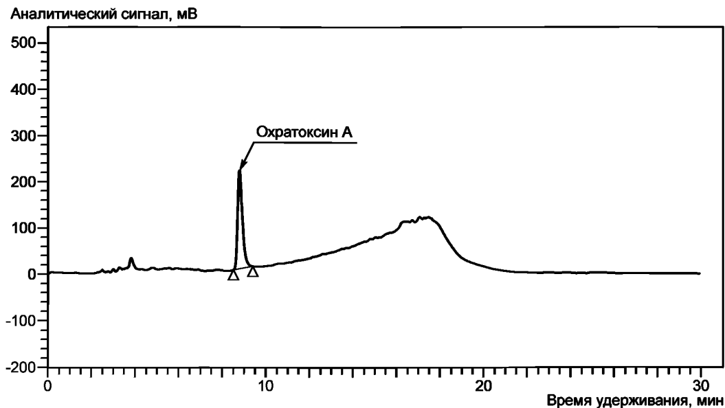
Рисунок А.1 — Хроматограмма пробы продукта для детского питания на зерновой основе, загрязненной охратоксином А естественным путем. Содержание охратоксина А 0,191 мкг/кг. Хроматограмма получена при межлабораторных испытаниях. Условия хроматографического анализа — по 7.1, градиентное элюирование
