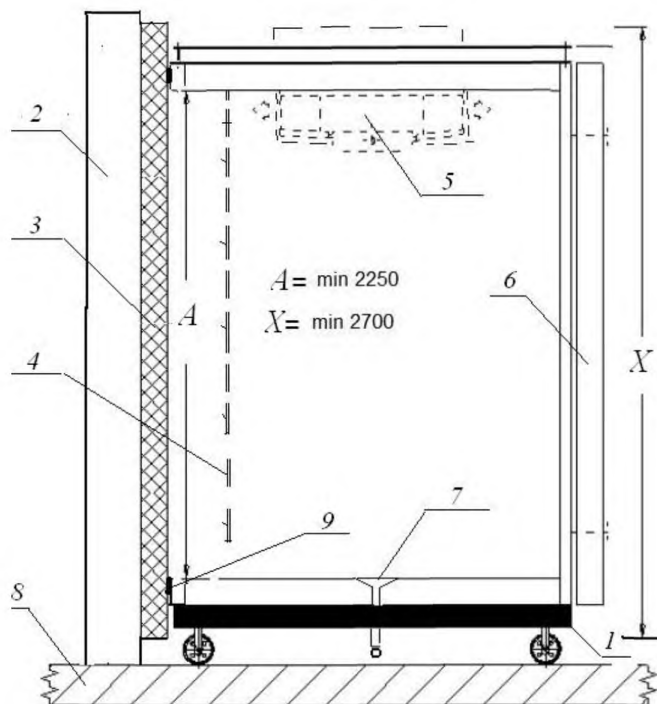
б) Внутренняя часть стенда (вид сбоку)
