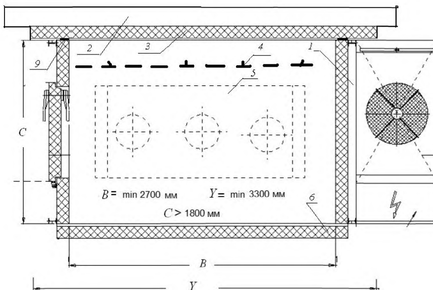
а) Внутренняя часть стенда (вид сверху)
