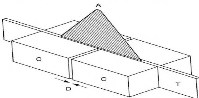
А — распределение деформации; С — зажимы; D — направление сжатия; Т — испытываемый образец
