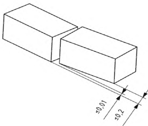
Рисунок А.1 — Расположение губок зажимов в горизонтальной плоскости
