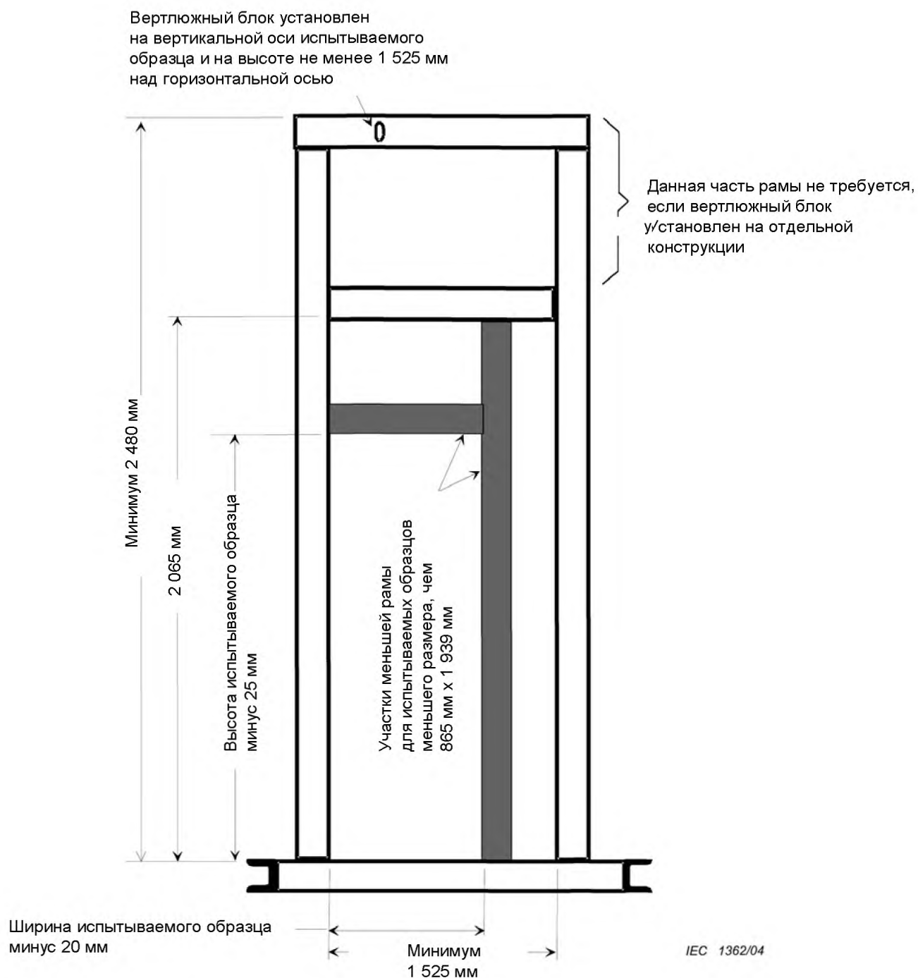
Рисунок 6 — Конструкция № 2 для испытания на удар
