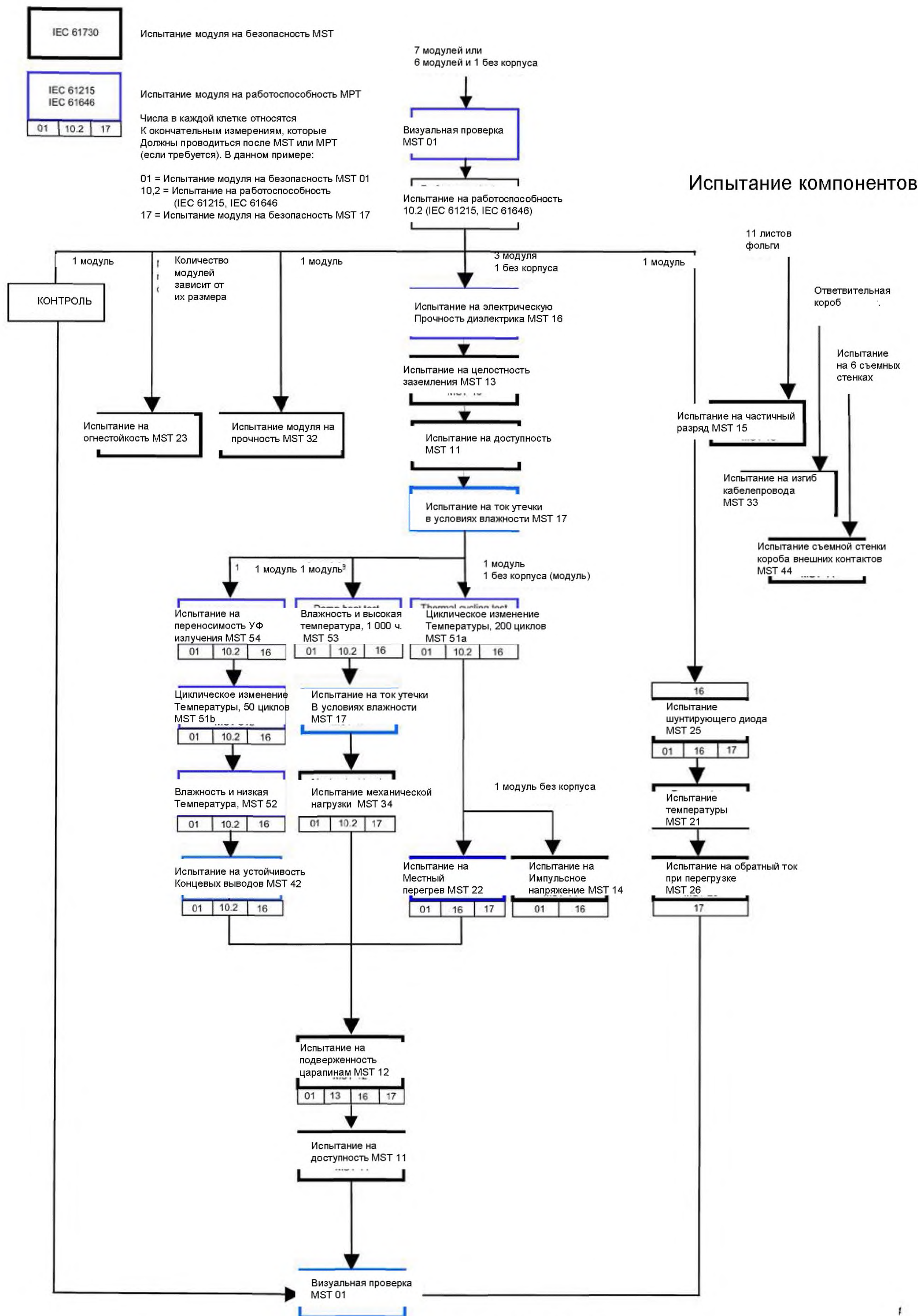
Рисунок 1 — Схма испытаний
