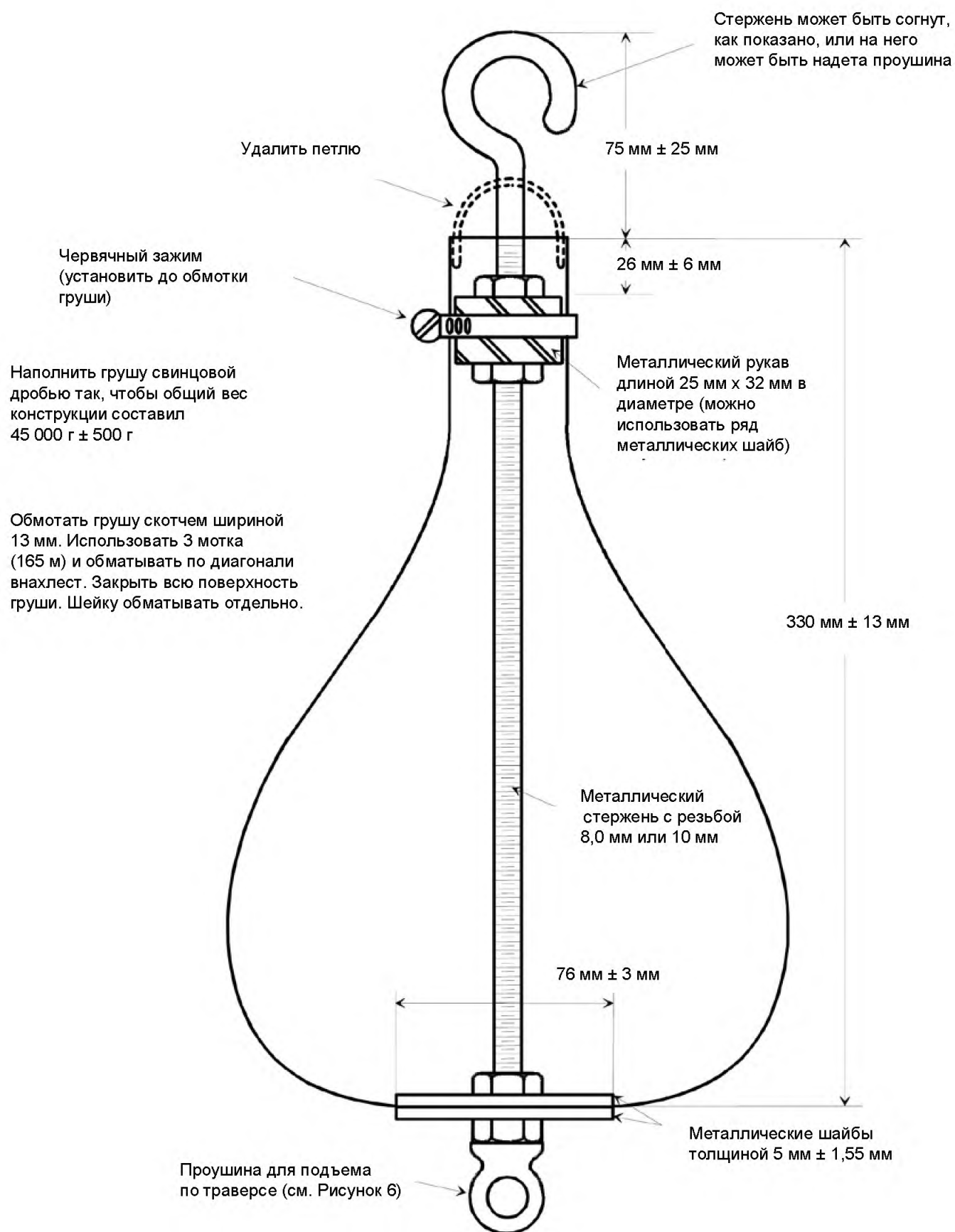
Рисунок 4 — Ударная груша
